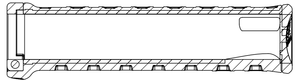
SCHNITT B-B
